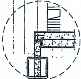
แบบขยาย 2
